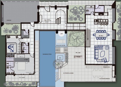
Первый этаж
